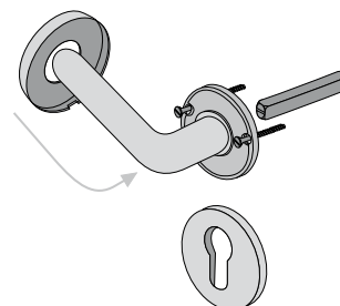
SOTTOROSSETTA IN METALLO - Ø 53 FERRO Ø 8 MM
